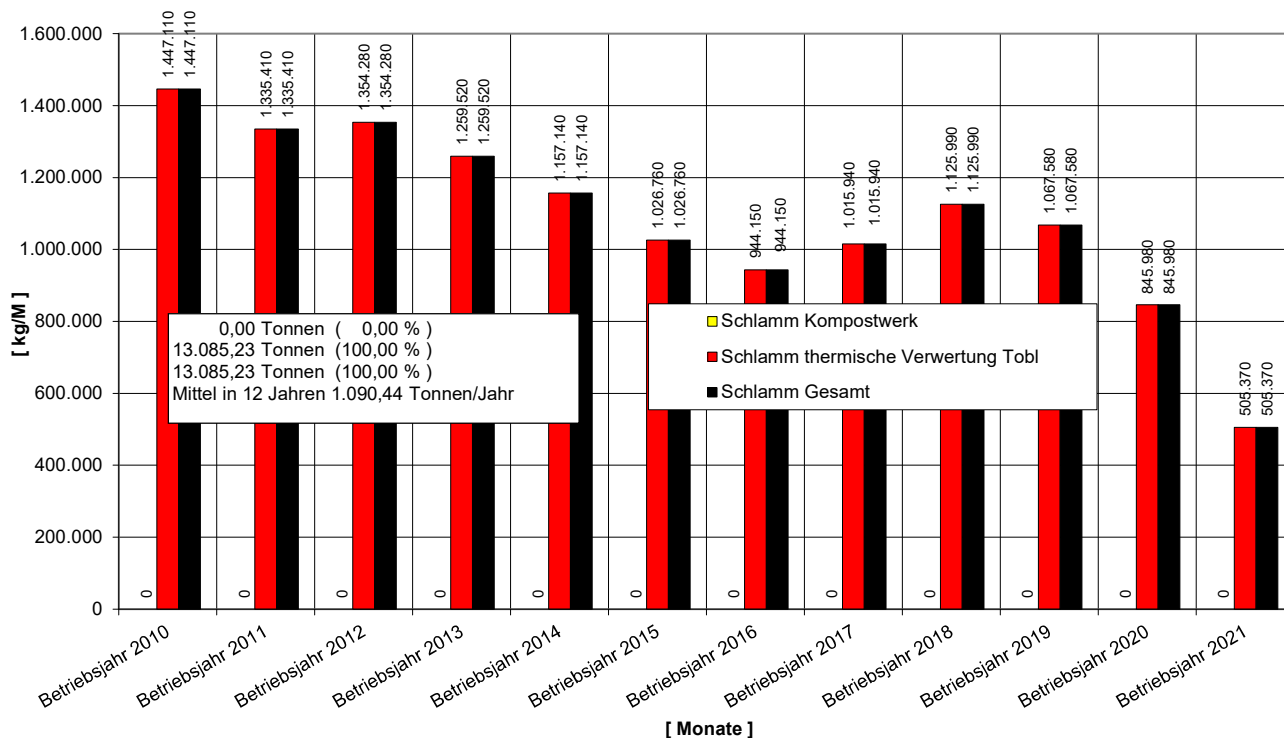
Schlammmanagement der Kläranlage Sompunt-Abtei; Betriebsjahre 2010-2021
