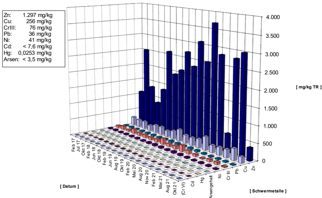
Schwermetalle im Schlamm in mg/kg TR; Kläranlage Sompunt; Betriebsjahre 2017-2021
