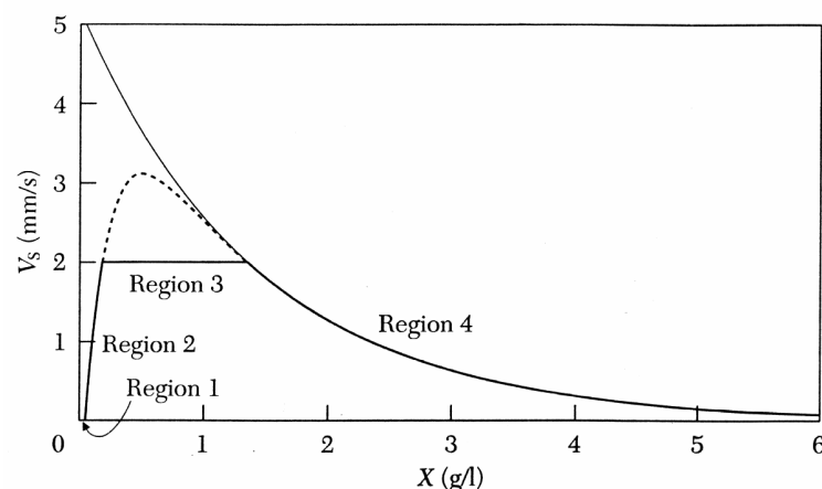
Abbildung 2.2: Sinkgeschwindigkeit nach Takács (entnommen Ekama et al. 1997)
