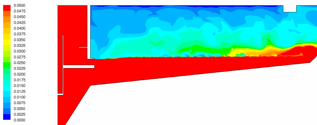
Abbildung 5.50: Schwebstoffverteilung [g/l] – Variante 1
