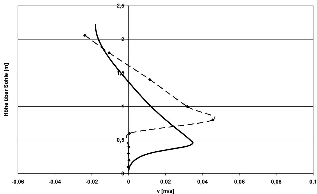
Abbildung 5.10: Vergleich von gemessenen und simulierten Horizontalgeschwindigkeiten – 10 m vom Einlauf
