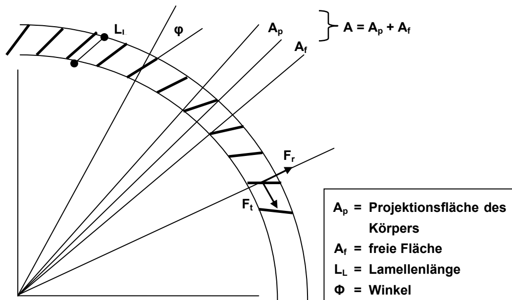
Abbildung 3.2: Lamellenkonstruktion im Einlauf eines Nachklärbeckens – Draufsicht
