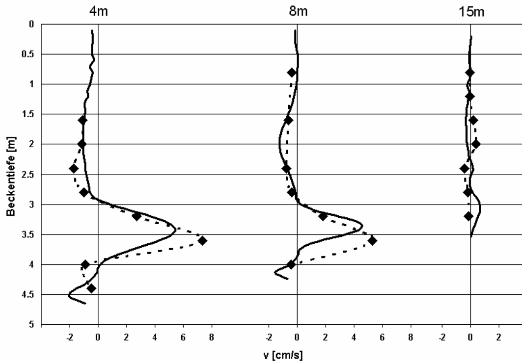
Abbildung 5.43: Vergleich von simulierten und gemessenen Horizontalgeschwindigkeiten
