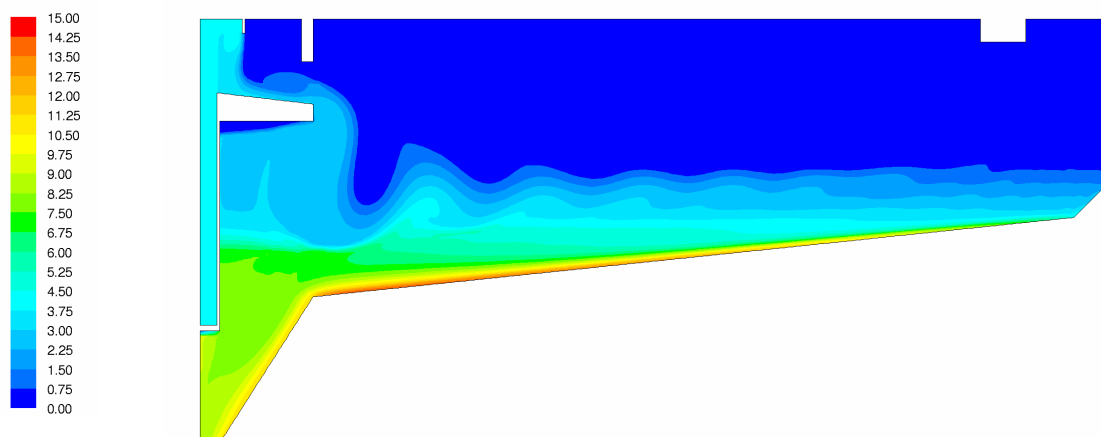
Abbildung 5.39: Schlammverteilung [g/l]
