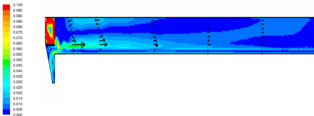
Abbildung 5.31: Geschwindigkeitsverteilung [m/s] – Optimierung
