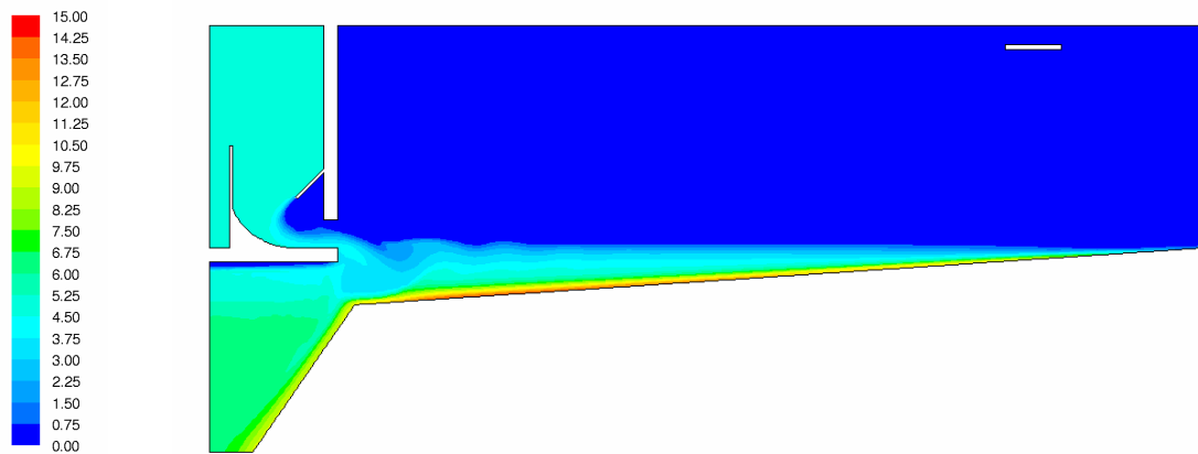
Abbildung 4.16: Schlammverteilung [g/l] - tiefer Einlauf
