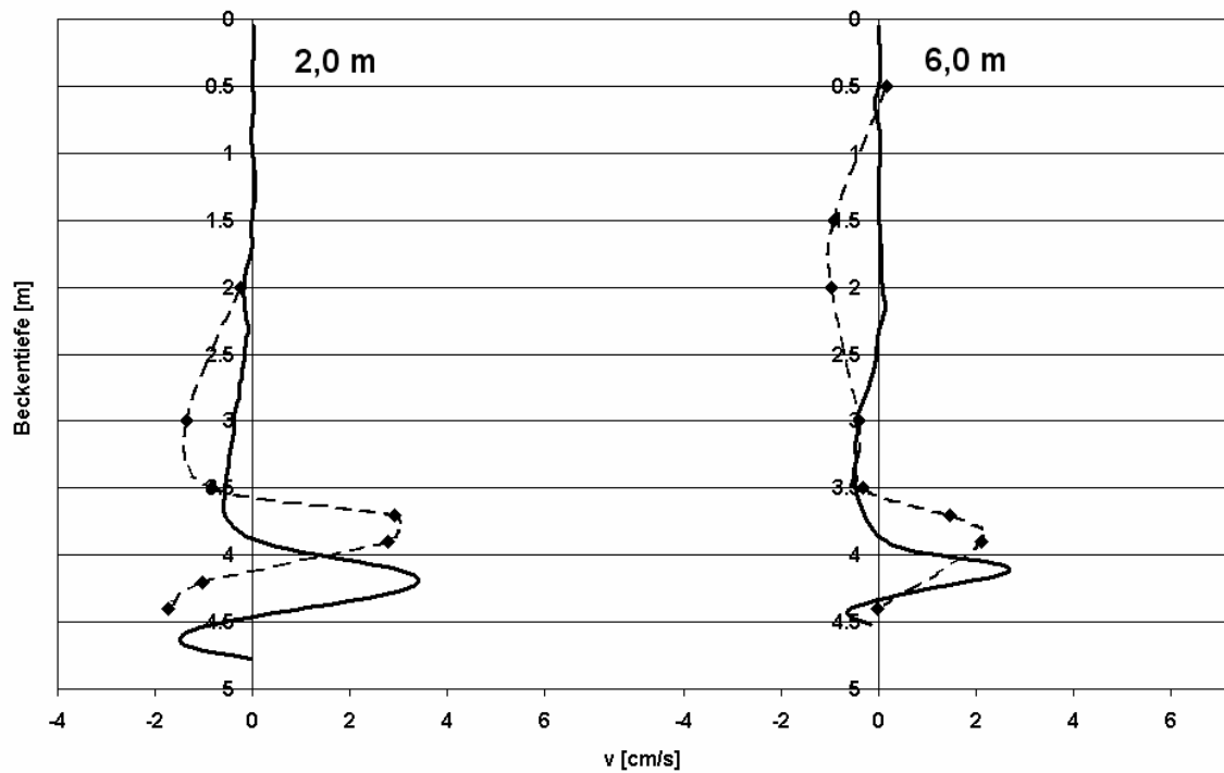
Abbildung 4.22: Vergleich von gemessenen und simulierten Radialgeschwindigkeiten – tiefer Einlauf – Lastfall 2
