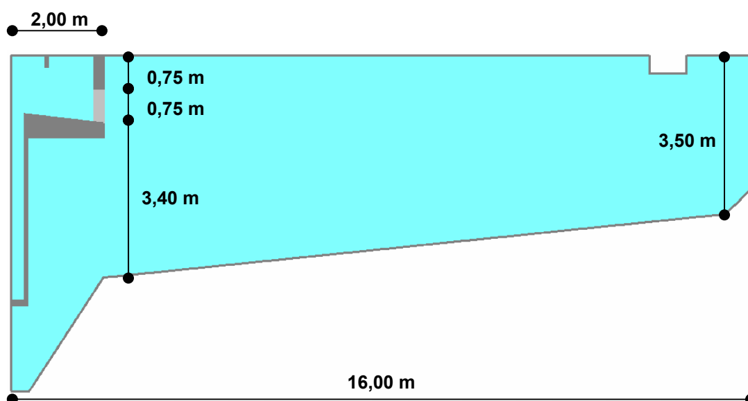
Abbildung 5.37: Querschnitt des Nachklärbeckens Miesbach
