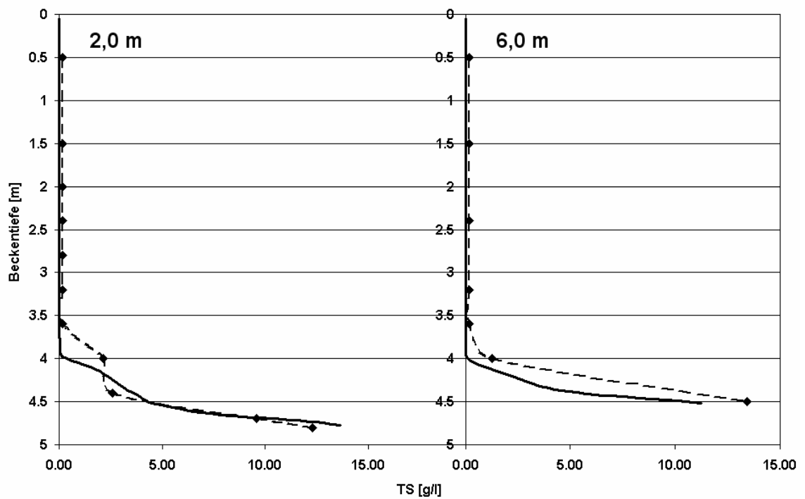
Abbildung 4.23: Vergleich von gemessenen und simulierten TS-Konzentrationen – tiefer Einlauf – Lastfall 2
