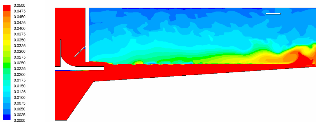
Abbildung 4.29: Schwebstoffverteilung [g/l] - optimierter Einlauf
