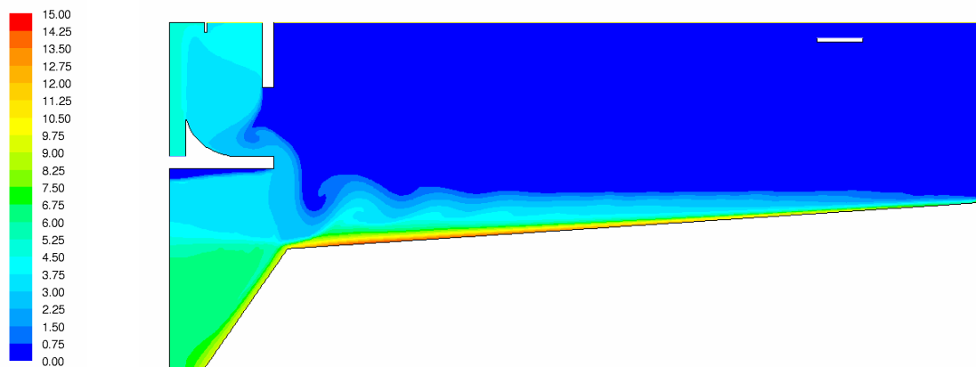
Abbildung 4.4: Schlammverteilung [g/l] - hoher Einlauf
