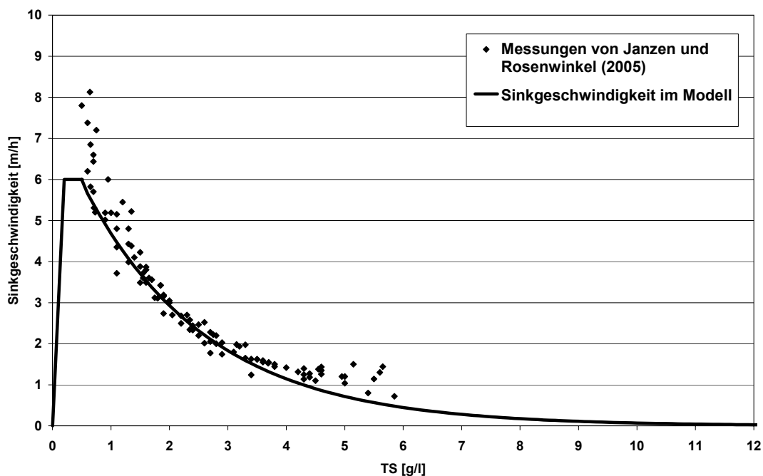
Abbildung 3.6: Absetzverhalten des Schlammes des Nachklärbeckens Rheda-Wiedenbrück
