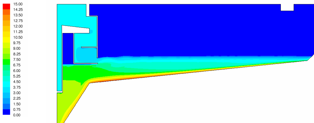
Abbildung 5.55: Schlammverteilung [g/l] – Variante 3
