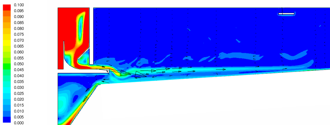
Abbildung 4.27: Geschwindigkeitsverteilung [m/s] - optimierter Einlauf
