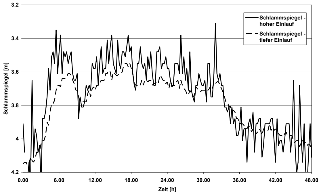
Abbildung 4.32: Gemessene Schlammбетhöhe
