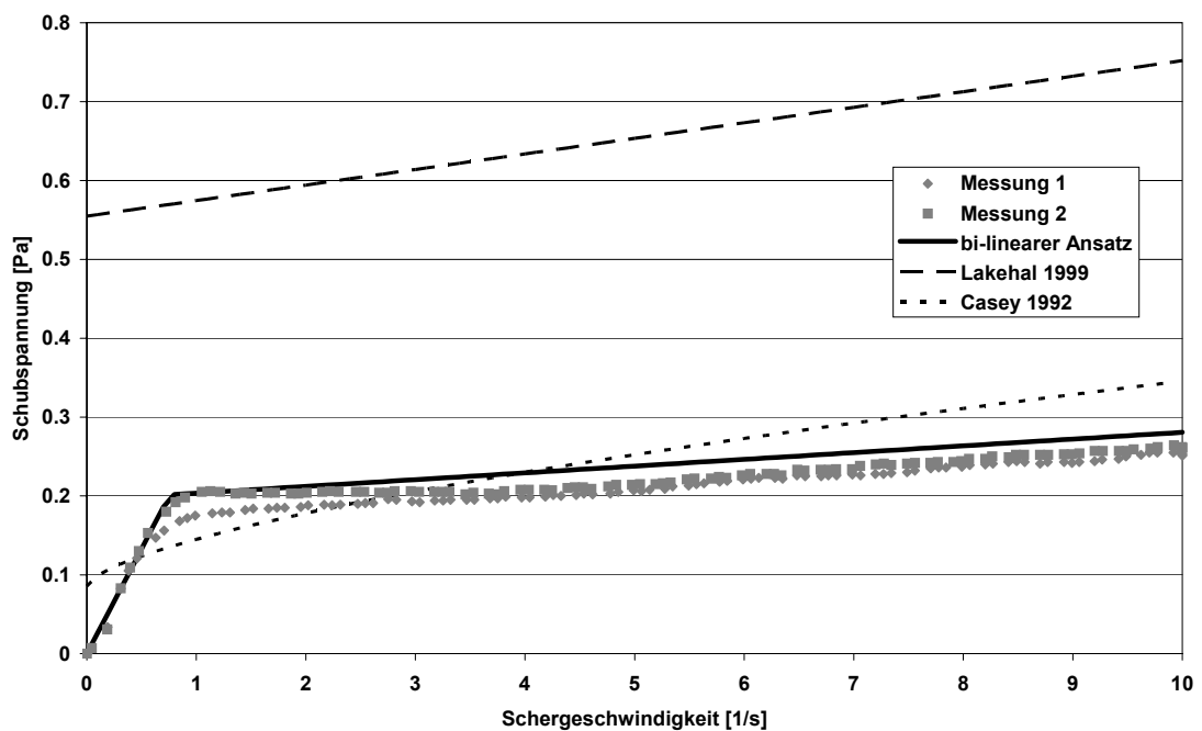
Abbildung 3.11: Schubspannungen bei einer TS-Konzentration von 8,7 g/l
