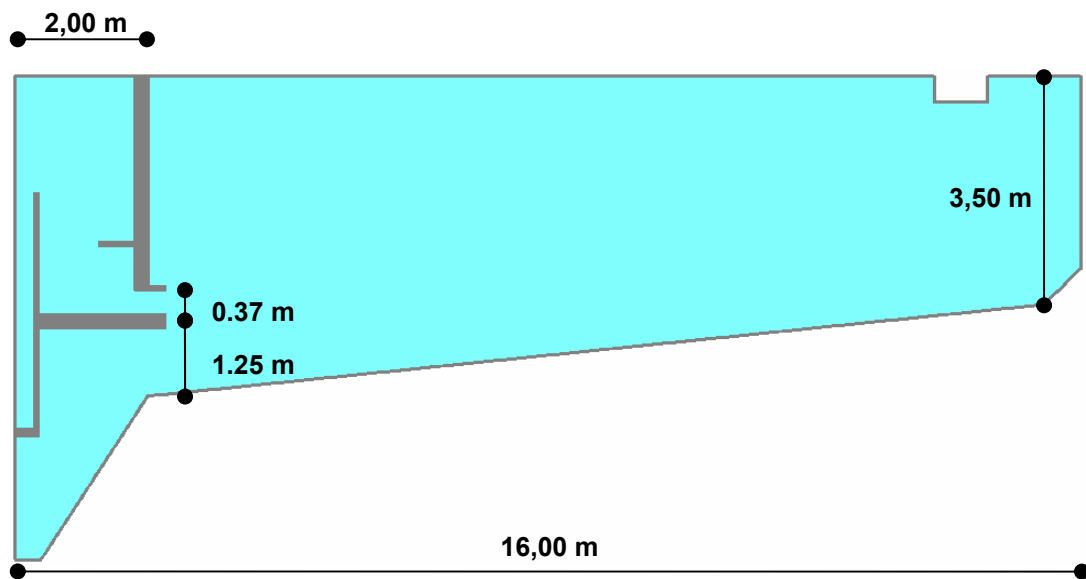
Abbildung 5.45: Querschnitt der Optimierungsvariante 1
