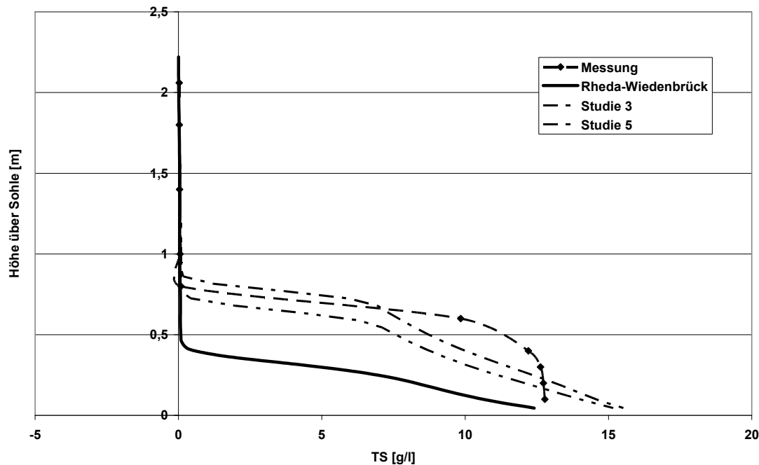
Abbildung 5.29: Vergleich der Feststoffverteilung in den einzelnen Parameterstudien – 10 m vom Einlauf entfernt
