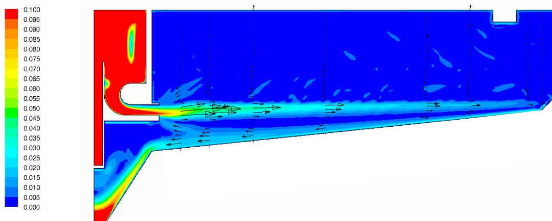
Abbildung 5.51: Geschwindigkeitsverteilung [m/s] – Variante 2
