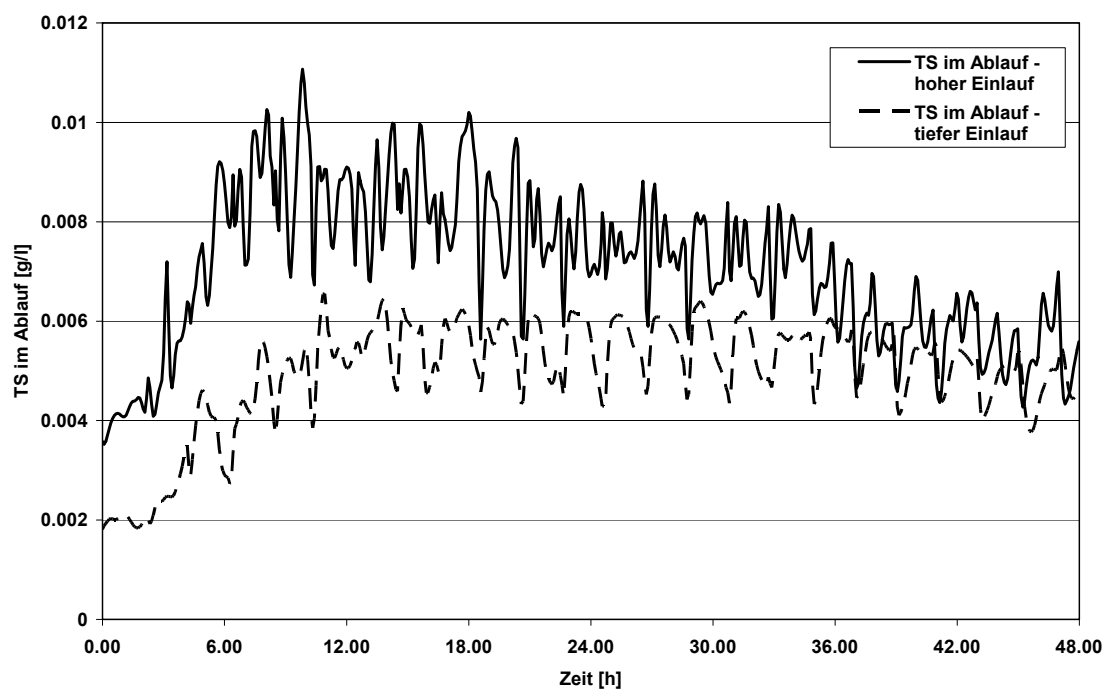
Abbildung 4.35: Simulierte TS-Konzentrationen im Ablauf der beiden Nachklärbecken
