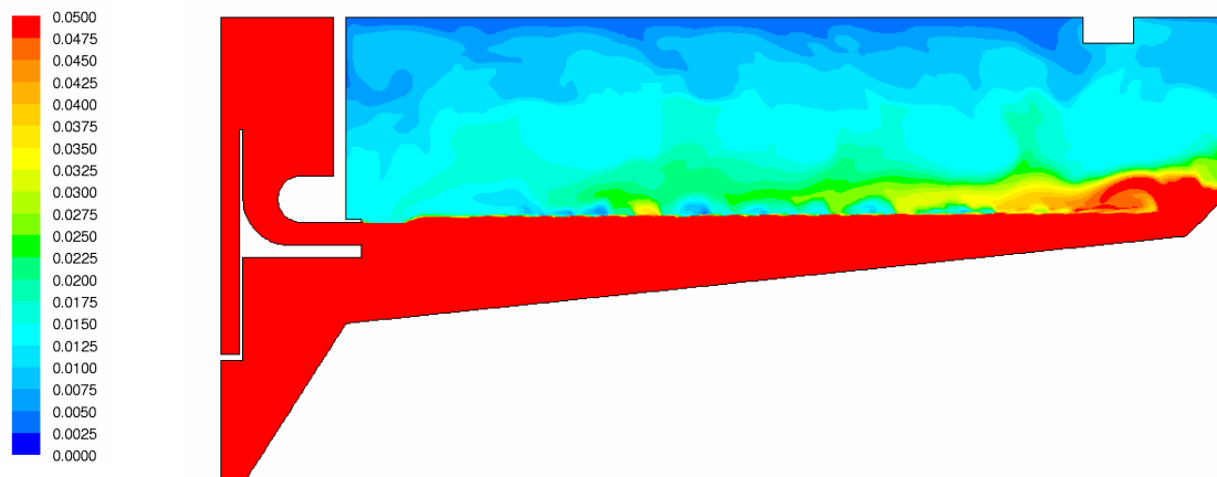
Abbildung 5.53: Schwebstoffverteilung [g/l] – Variante 2
