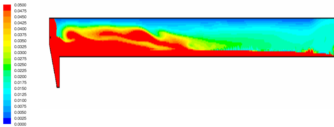
Abbildung 5.5: Schwebstoffverteilung [g/l]
