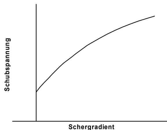
Abbildung 2.6: Fließkurve für ein Herschel-Bulkley-Fluid
