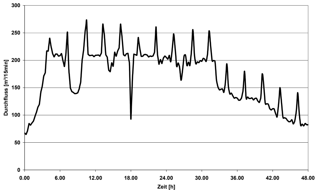
Abbildung 4.30: Zulaufganglinie zur Belebung
