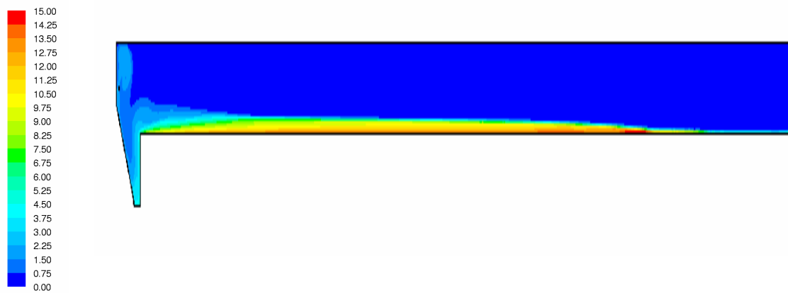
Abbildung 5.16: Schlammverteilung [g/l] – Studie 1
