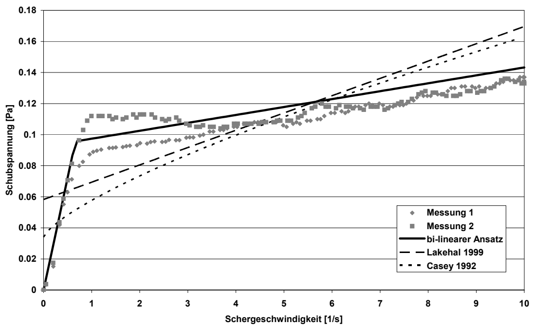
Abbildung 3.10: Schubspannungen bei einer TS-Konzentration von 6,4 g/l
