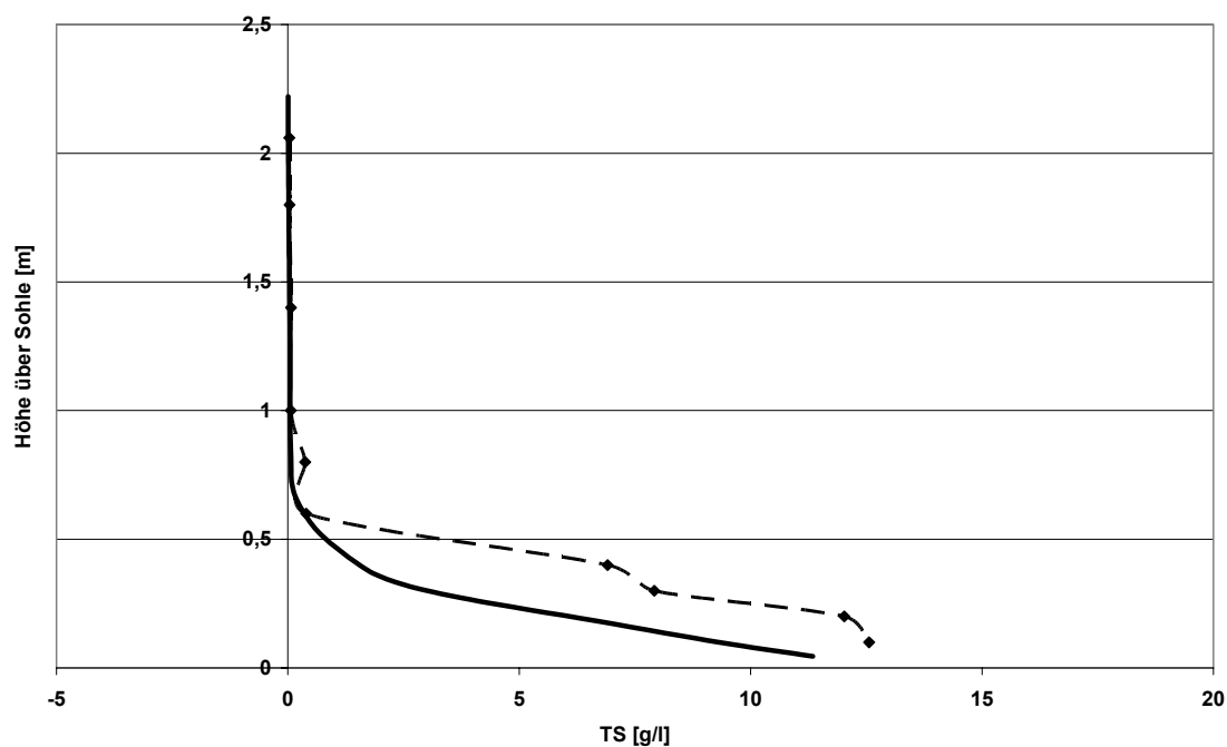
Abbildung 5.9: Vergleich von gemessener und simulierter Feststoffverteilung – 5 m vom Einlauf
