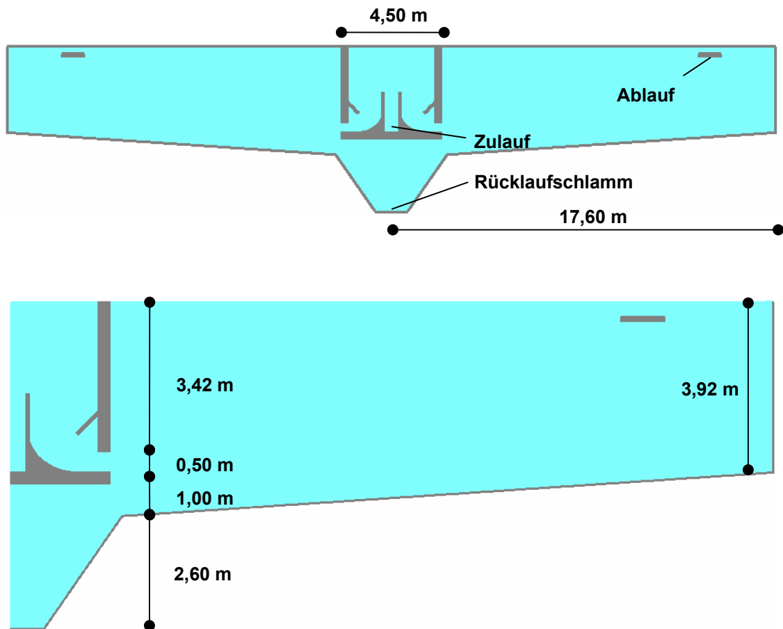
Abbildung 4.2: Querschnitt des Nachklärbeckens Rheda-Wiedenbrück mit tiefem Einlauf
