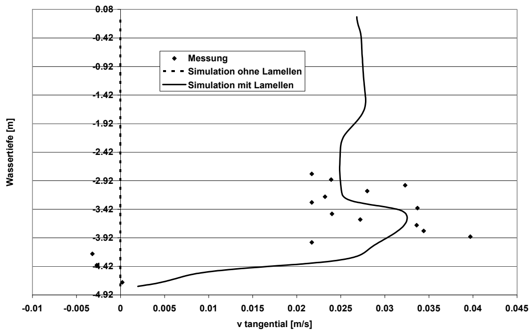
Abbildung 3.4: Tangentialgeschwindigkeiten in einem Profil 2m vom Einlauf entfernt
