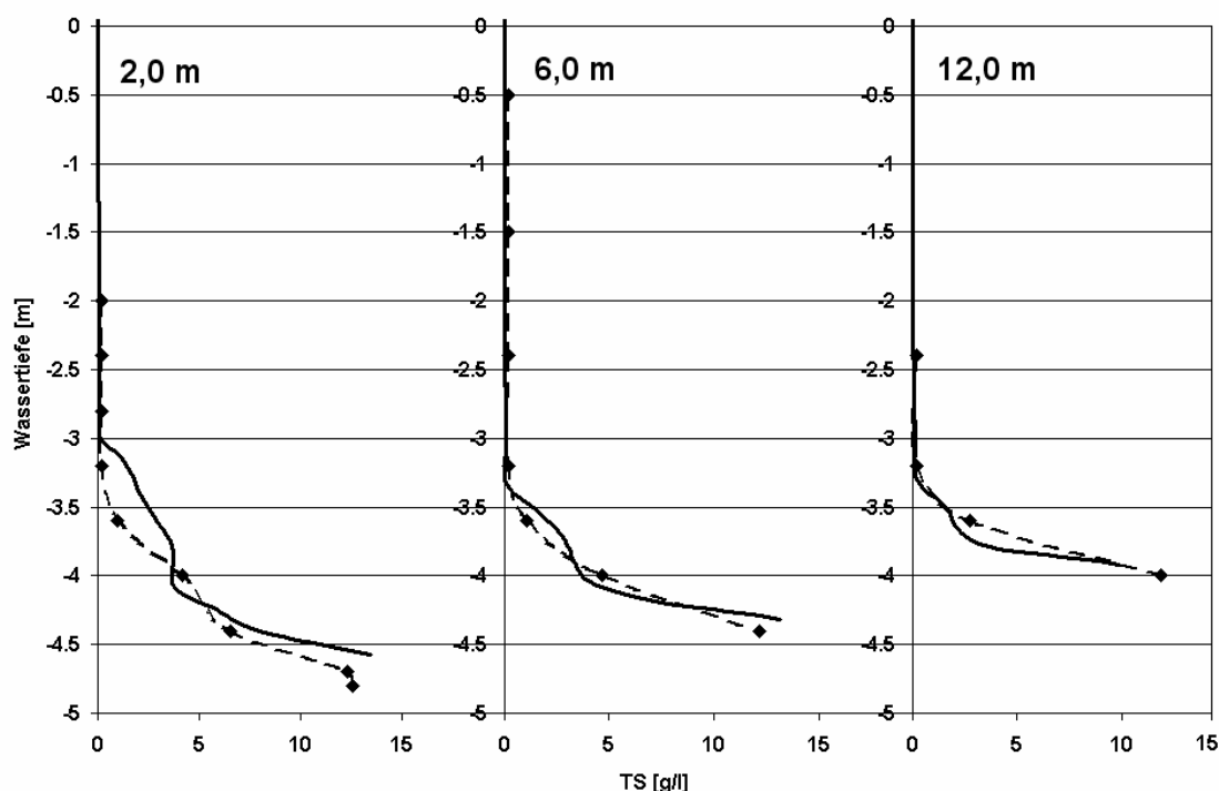
Abbildung 4.10: Vergleich von gemessenen und simulierten TS-Konzentrationen – hoher Einlauf – Lastfall 1
