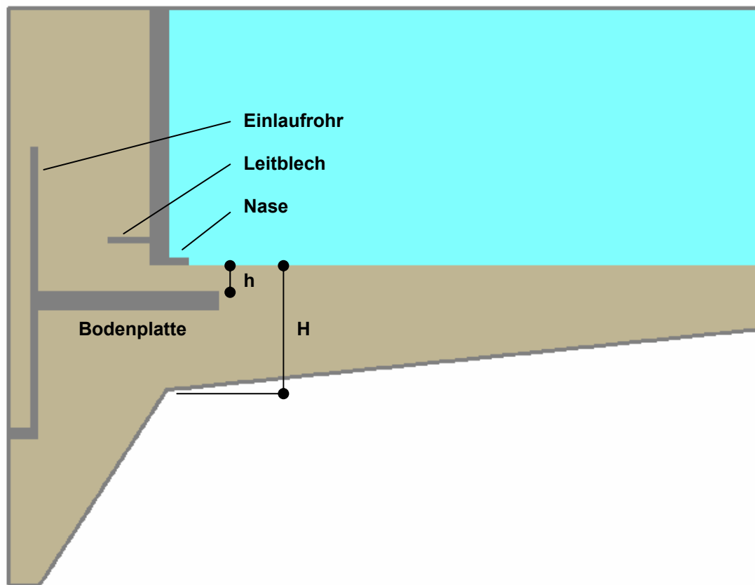
Abbildung 6.1: Empfehlungen für die Konstruktion des Einlaufbauwerkes
