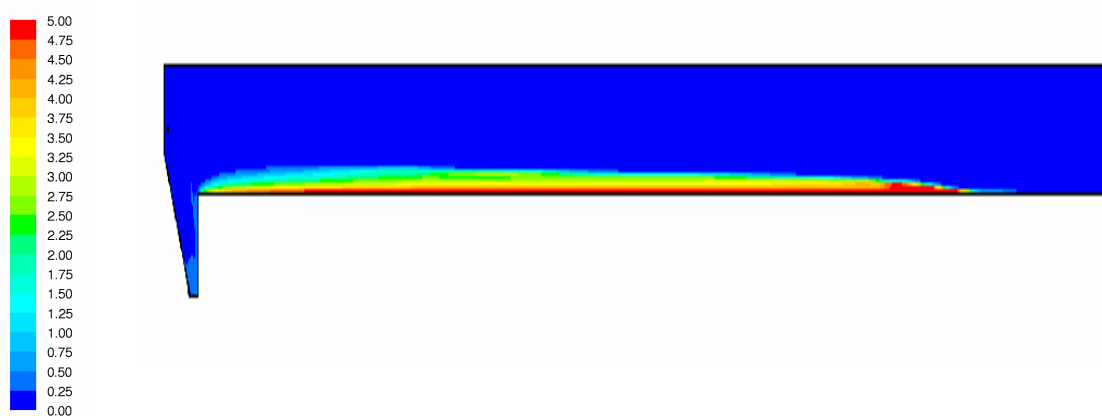
Abbildung 5.27: Verteilung der Viskosität [\text{Ns/m}^2] – Studie 6
