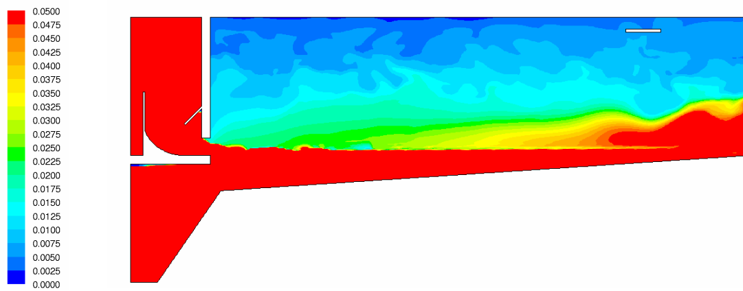
Abbildung 4.17: Schwebstoffverteilung [g/l] - tiefer Einlauf
