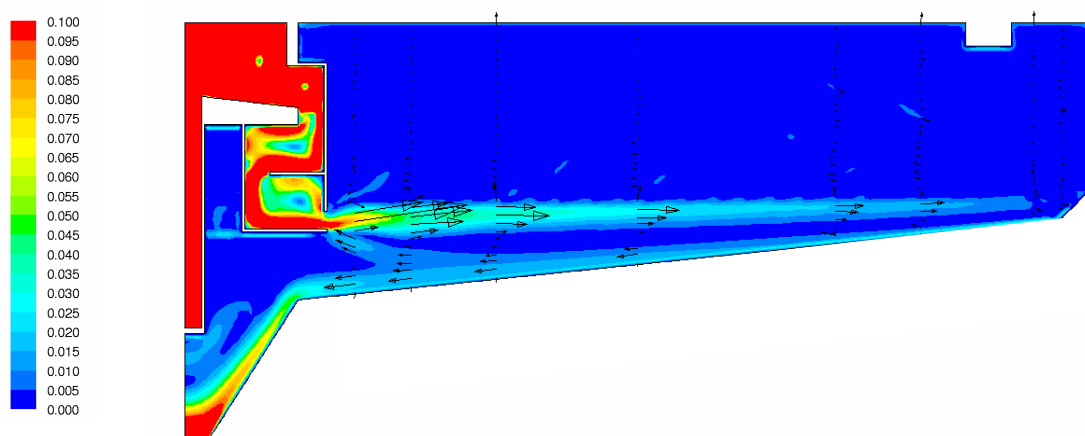
Abbildung 5.54: Geschwindigkeitsverteilung [m/s] – Variante 3
