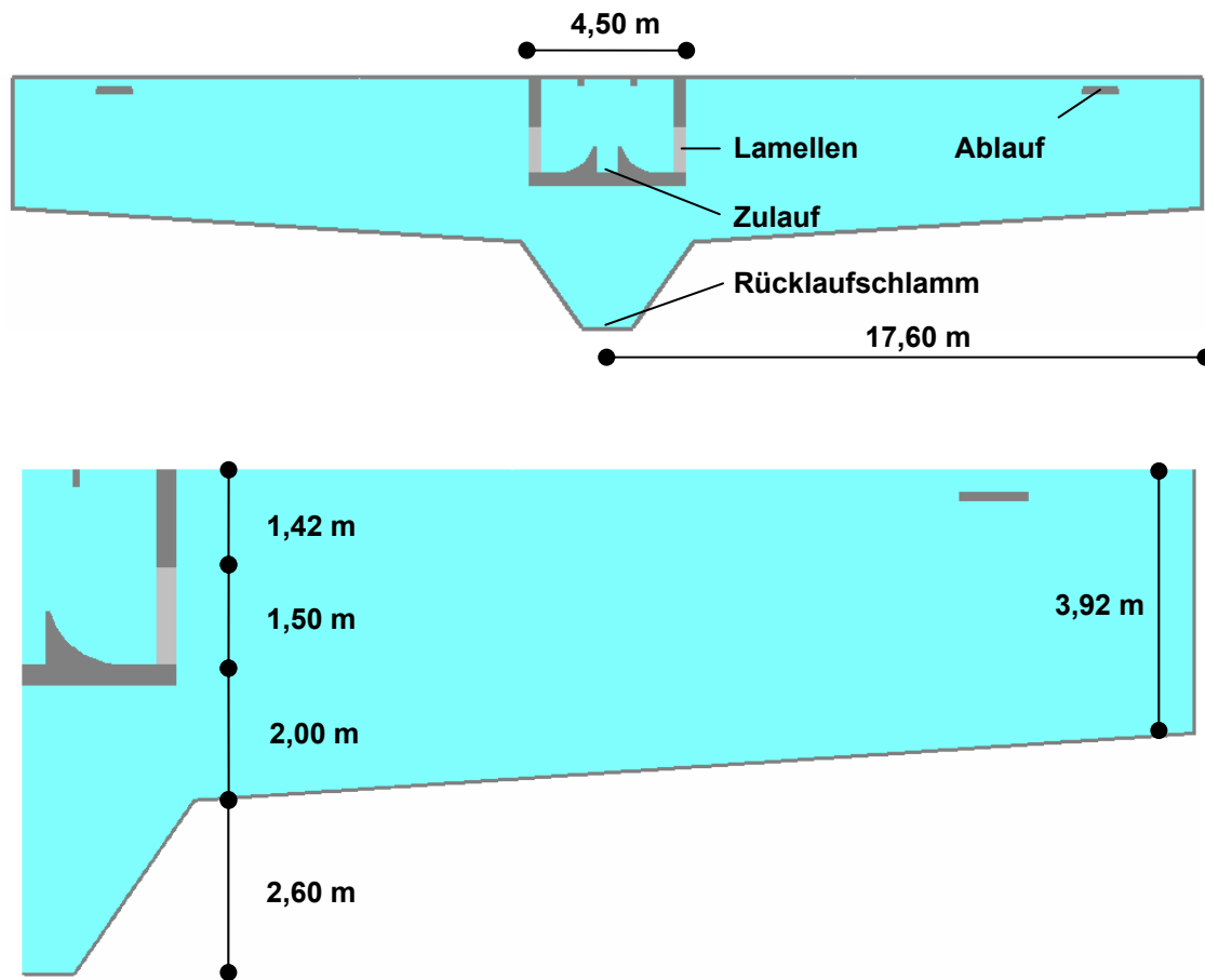
Abbildung 4.1: Querschnitt des Nachklärbeckens Rheda-Wiedenbrück mit hohem Einlauf
