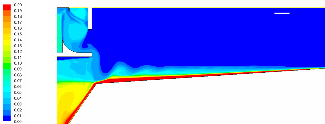
Abbildung 4.7: Verteilung der Viskosität [Ns/m^2] - hoher Einlauf
