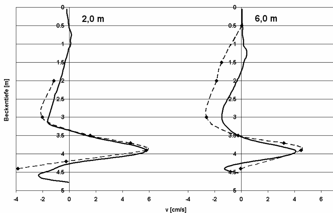
Abbildung 4.11: Vergleich von gemessenen und simulierten Radialgeschwindigkeiten – hoher Einlauf – Lastfall 2
