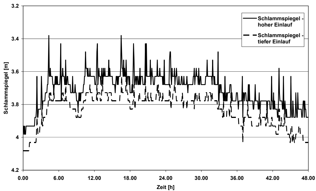
Abbildung 4.34: Simulierte Schlammбетhöhe
