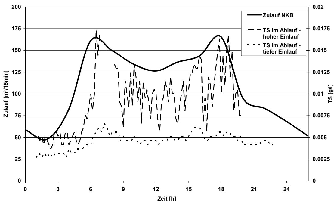
Abbildung 4.33: Gemessene TS-Konzentrationen im Ablauf der beiden Nachklärbecken bei einem vergleichbaren Regenereignis
