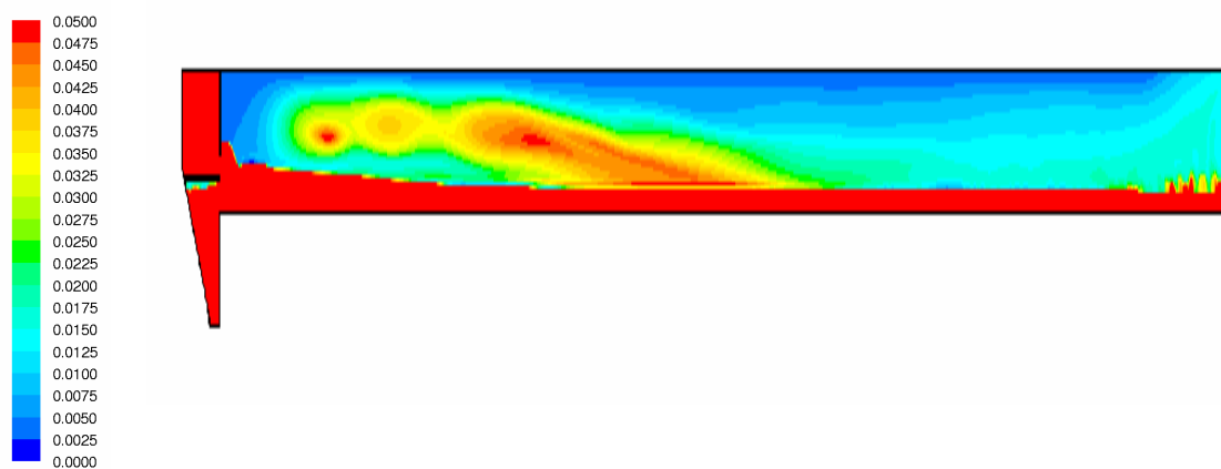
Abbildung 5.34: Schwebstoffverteilung [g/l] – Optimierung
