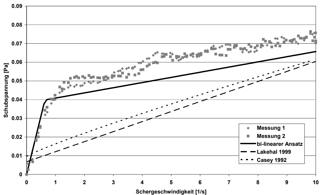
Abbildung 3.9: Schubspannungen bei einer TS-Konzentration von 4,2 g/l
