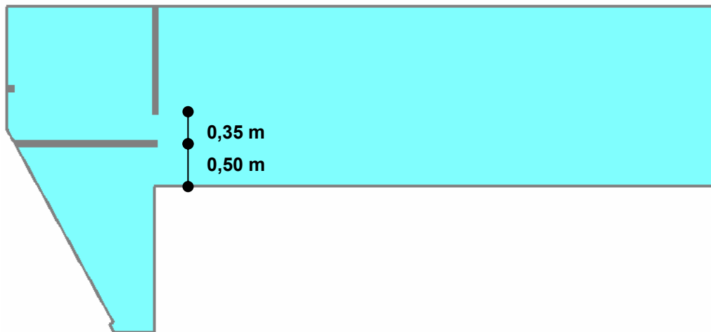
Abbildung 5.30: Geometrie der Einlaufoptimierung nach Krebs (2001)
