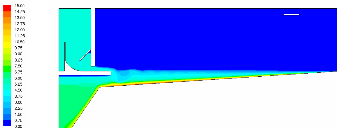
Abbildung 4.28: Schlammverteilung [g/l] - optimierter Einlauf
