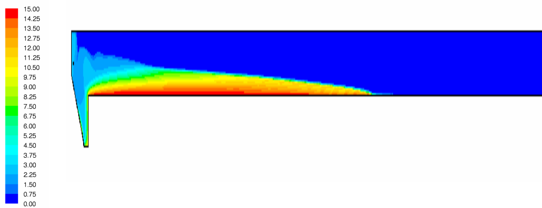
Abbildung 5.22: Schlammverteilung [g/l] – Studie 4
