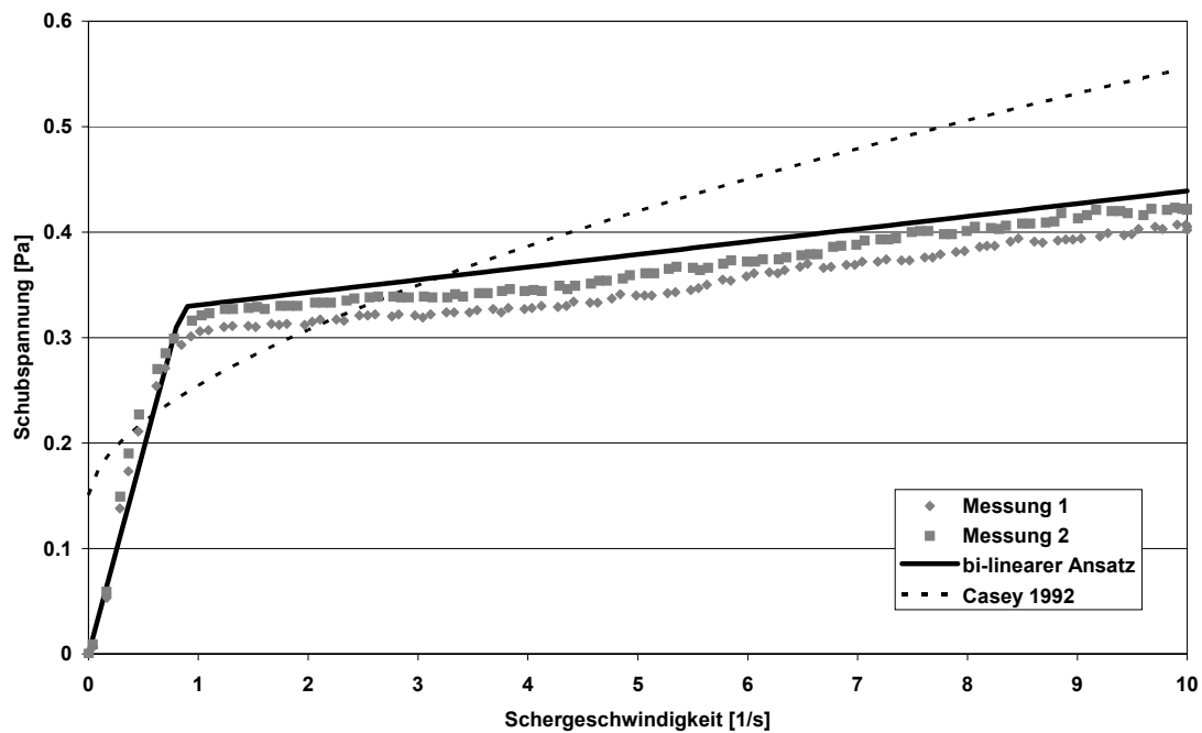
Abbildung 3.12: Schubspannungen bei einer TS-Konzentration von 10,5 g/l
