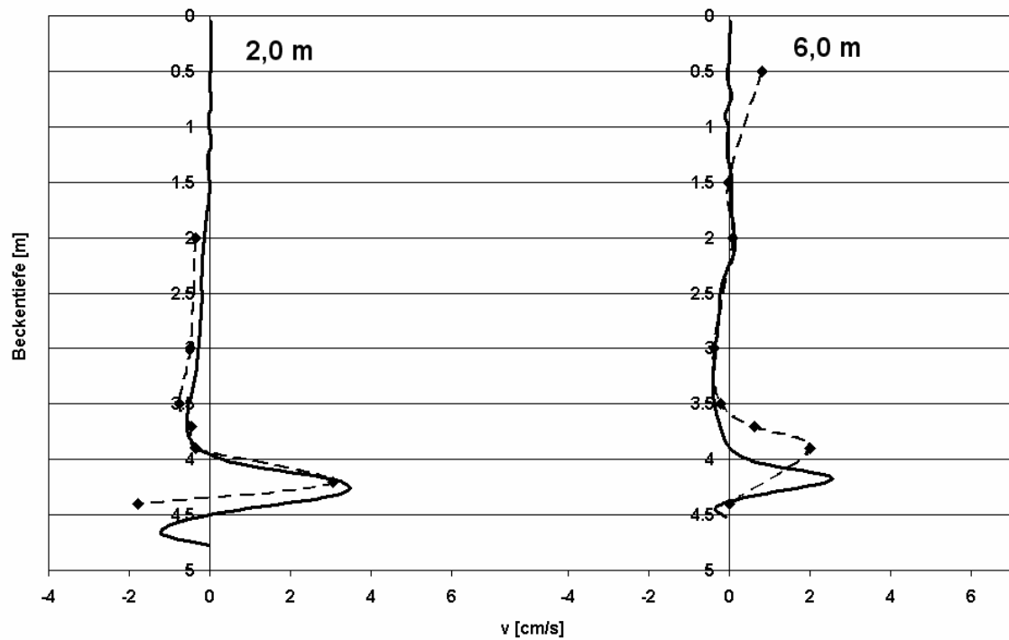
Abbildung 4.24: Vergleich von gemessenen und simulierten Radialgeschwindigkeiten – tiefer Einlauf – Lastfall 3
