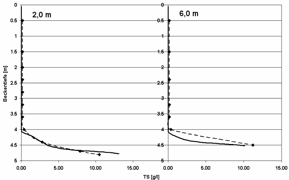
Abbildung 4.25: Vergleich von gemessenen und simulierten TS-Konzentrationen – tiefer Einlauf – Lastfall 3
