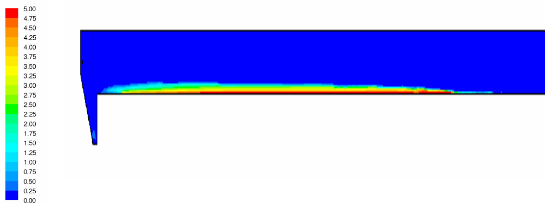
Abbildung 5.17: Verteilung der Viskosität [Ns/m²] – Studie 1
