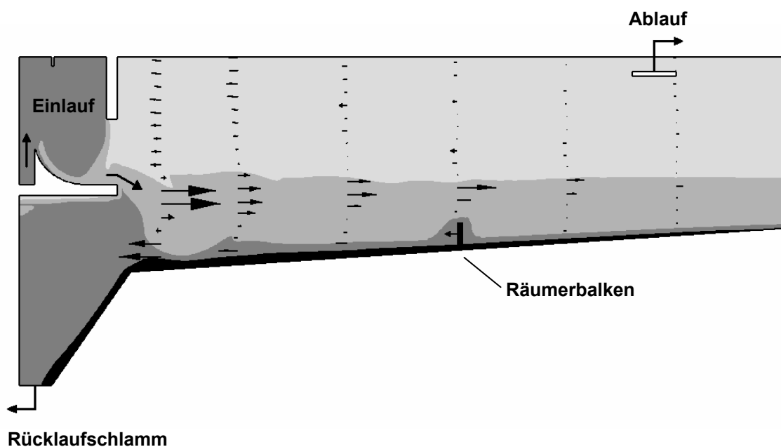
Abbildung 2.1: Grundlegendes Strömungsfeld in Nachklärbecken
