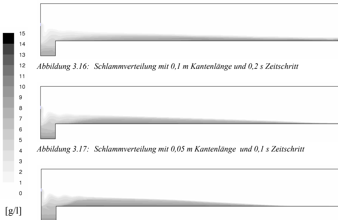
Abbildung 3.18: Schlammverteilung mit 0,025 m Kantenlänge und 0,05 s Zeitschritt
