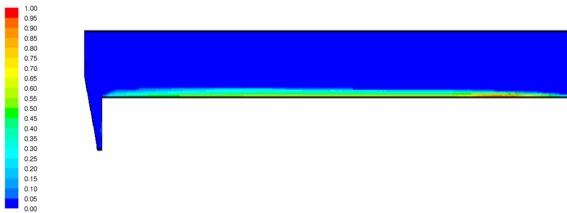
Abbildung 5.7: Verteilung der Viskosität [\text{Ns/m}^2]
