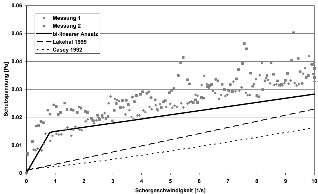
Abbildung 3.8: Schubspannungen bei einer TS-Konzentration von 2,2 g/l
