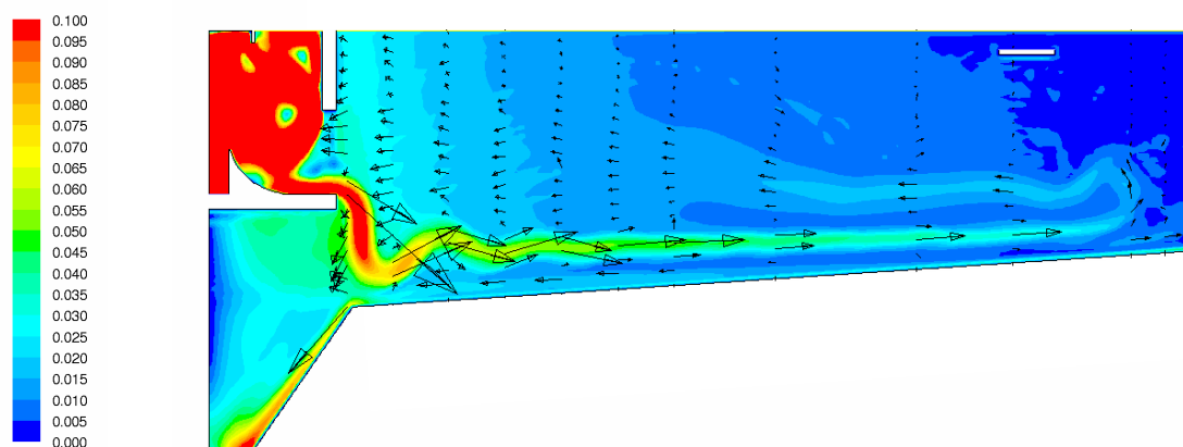
Abbildung 4.3: Geschwindigkeitsverteilung [m/s] - hoher Einlauf
