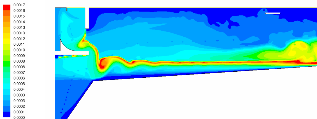
Abbildung 4.6: Verteilung der Sinkgeschwindigkeit [m/s] - hoher Einlauf
