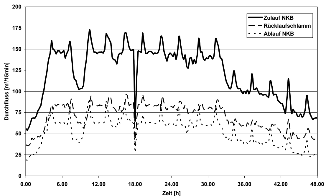
Abbildung 4.31: Resultierende Ganglinien für ein Nachklärbecken
