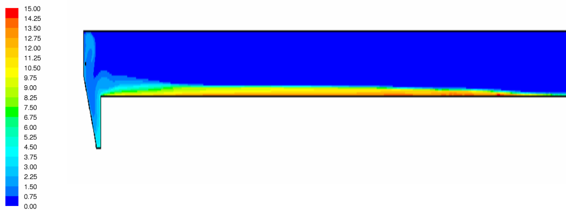
Abbildung 5.18: Schlammverteilung [g/l] – Studie 2
