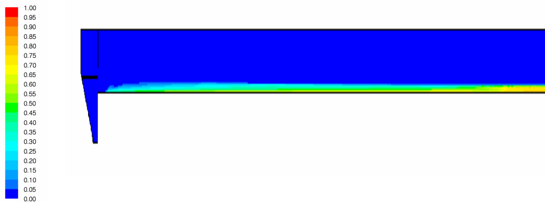
Abbildung 5.36: Verteilung der Viskosität [Ns/m²] – Optimierung
