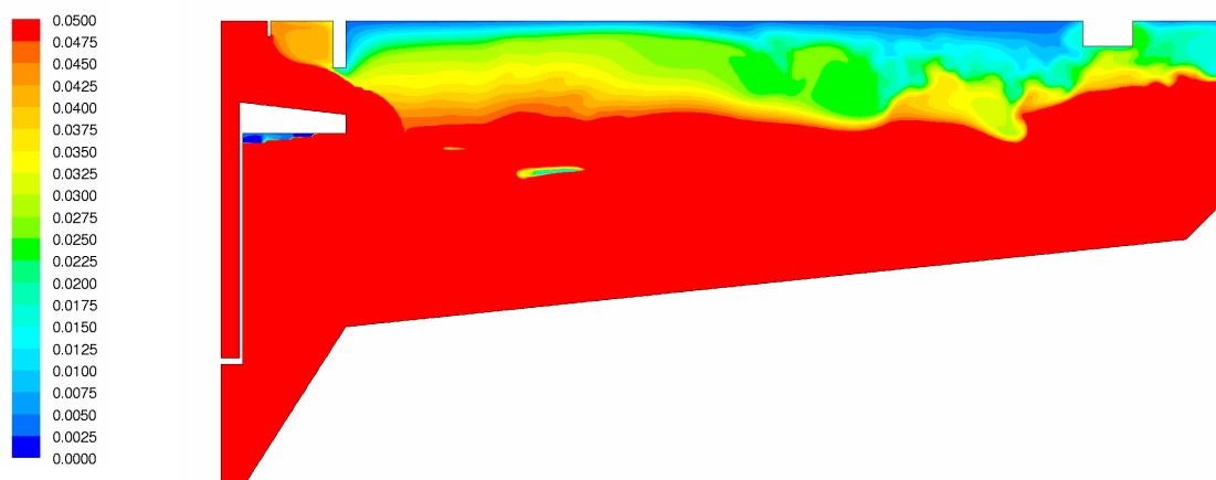
Abbildung 5.40: Schwebstoffverteilung [g/l]
