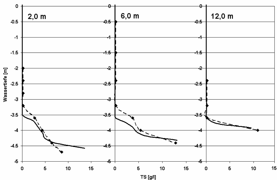
Abbildung 4.21: Vergleich von gemessenen und simulierten TS-Konzentrationen – tiefer Einlauf – Lastfall 1
