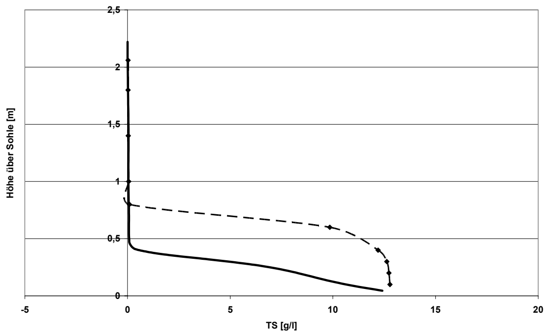
Abbildung 5.11: Vergleich von gemessener und simulierter Feststoffverteilung – 10 m vom Einlauf
