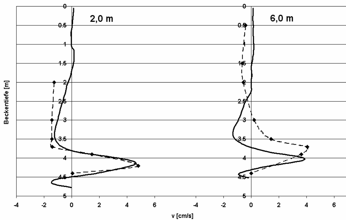
Abbildung 4.13: Vergleich von gemessenen und simulierten Radialgeschwindigkeiten – hoher Einlauf – Lastfall 3
