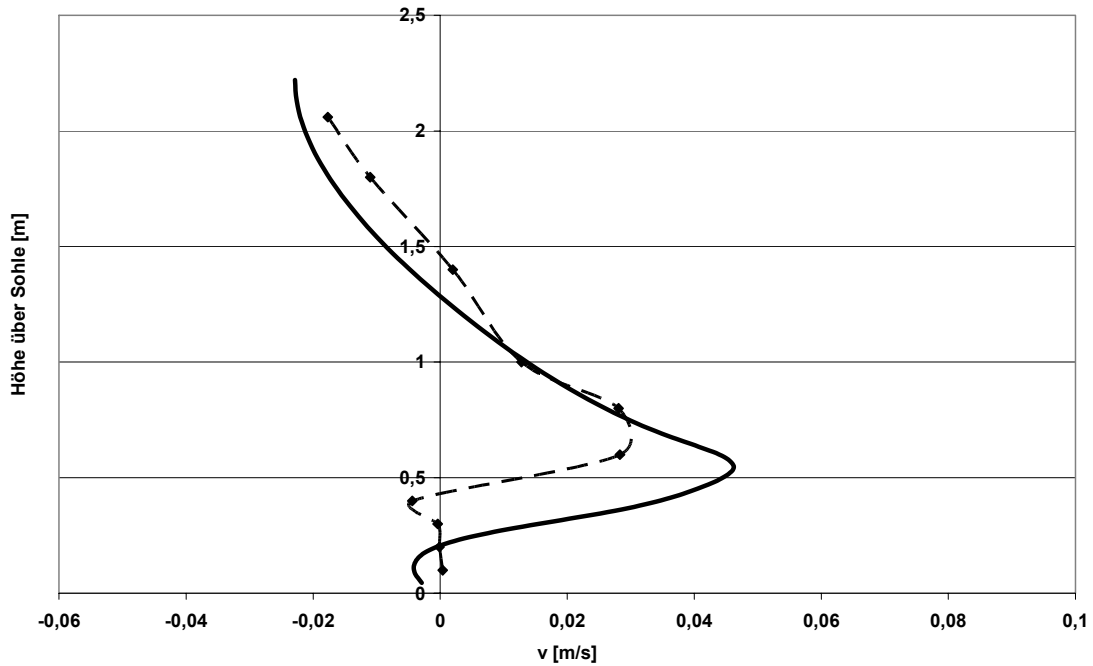
Abbildung 5.8: Vergleich von gemessenen und simulierten Horizontalgeschwindigkeiten – 5 m vom Einlauf
