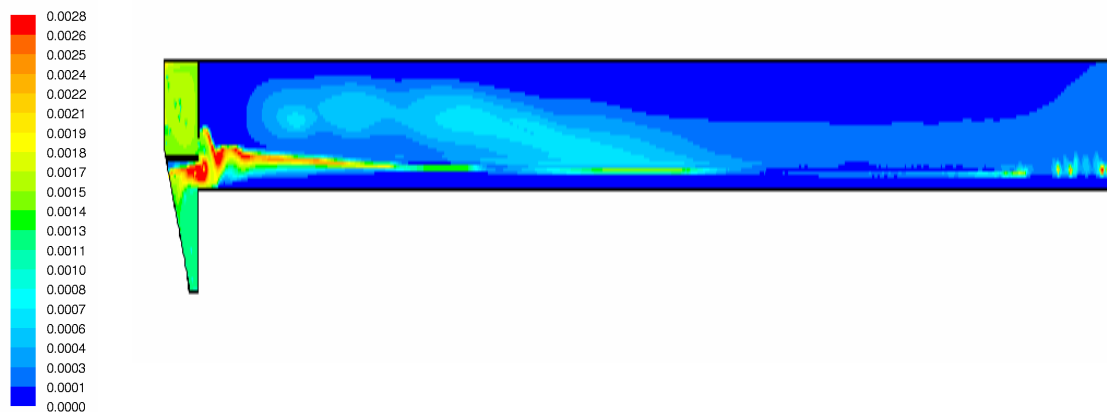
Abbildung 5.35: Verteilung der Sinkgeschwindigkeit [m/s] – Optimierung
