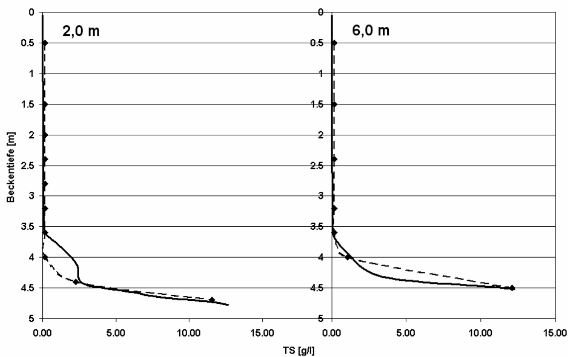
Abbildung 4.12: Vergleich von gemessenen und simulierten TS-Konzentrationen – hoher Einlauf – Lastfall 2
