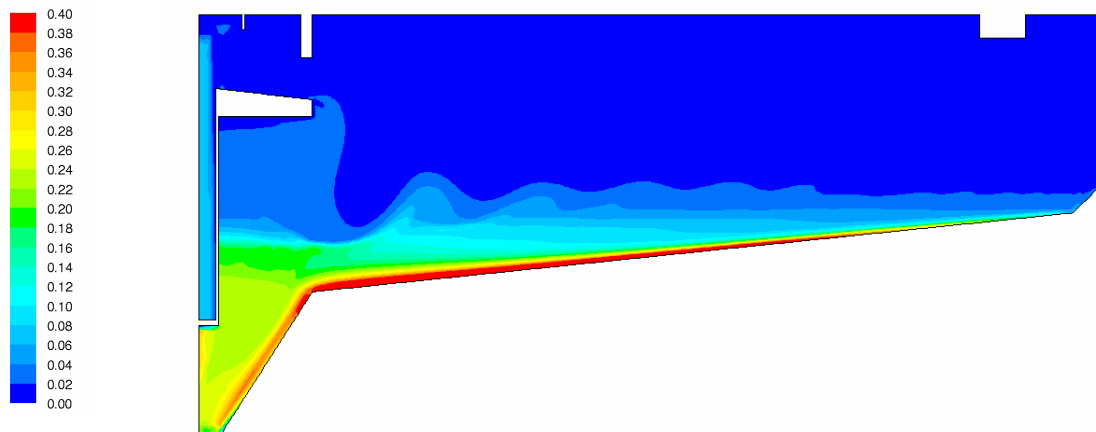
Abbildung 5.42: Verteilung der Viskosität [\text{Ns/m}^2]
