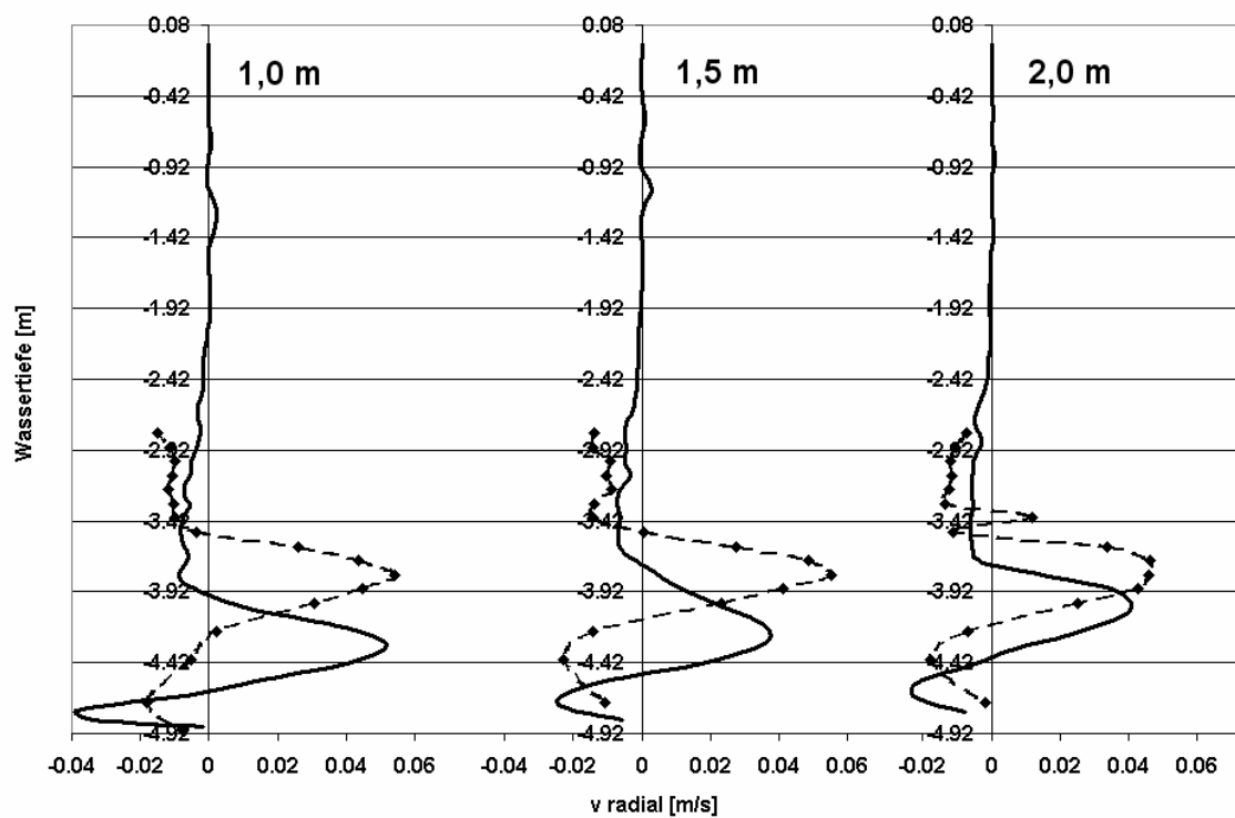
Abbildung 4.20: Vergleich von gemessenen und simulierten Radialgeschwindigkeiten – tiefer Einlauf – Lastfall 1
