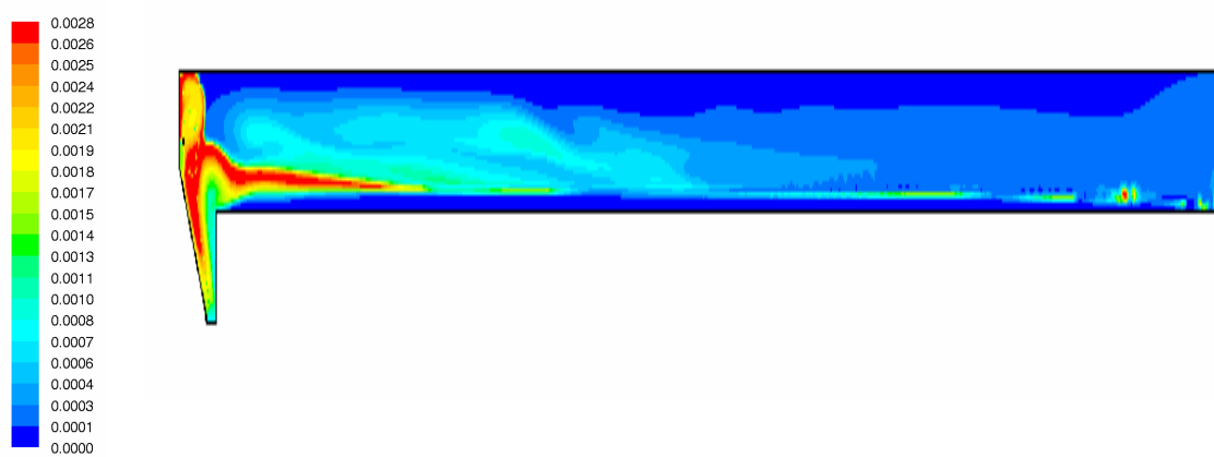
Abbildung 5.6: Verteilung der Sinkgeschwindigkeit [m/s]
