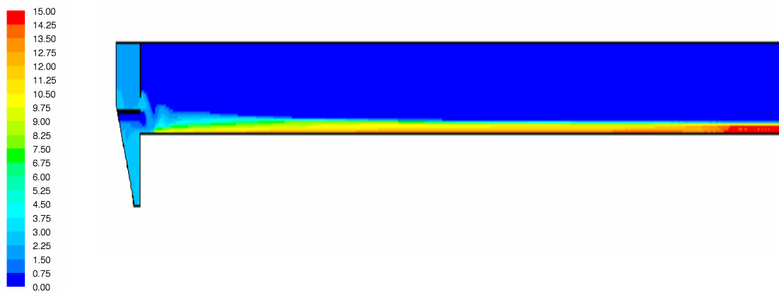
Abbildung 5.33: Schlammverteilung [g/l] – Optimierung
