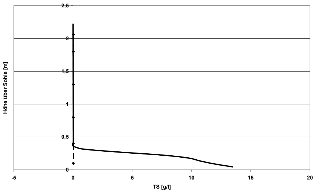
Abbildung 5.15: Vergleich von gemessener und simulierter Feststoffverteilung – 30 m vom Einlauf
