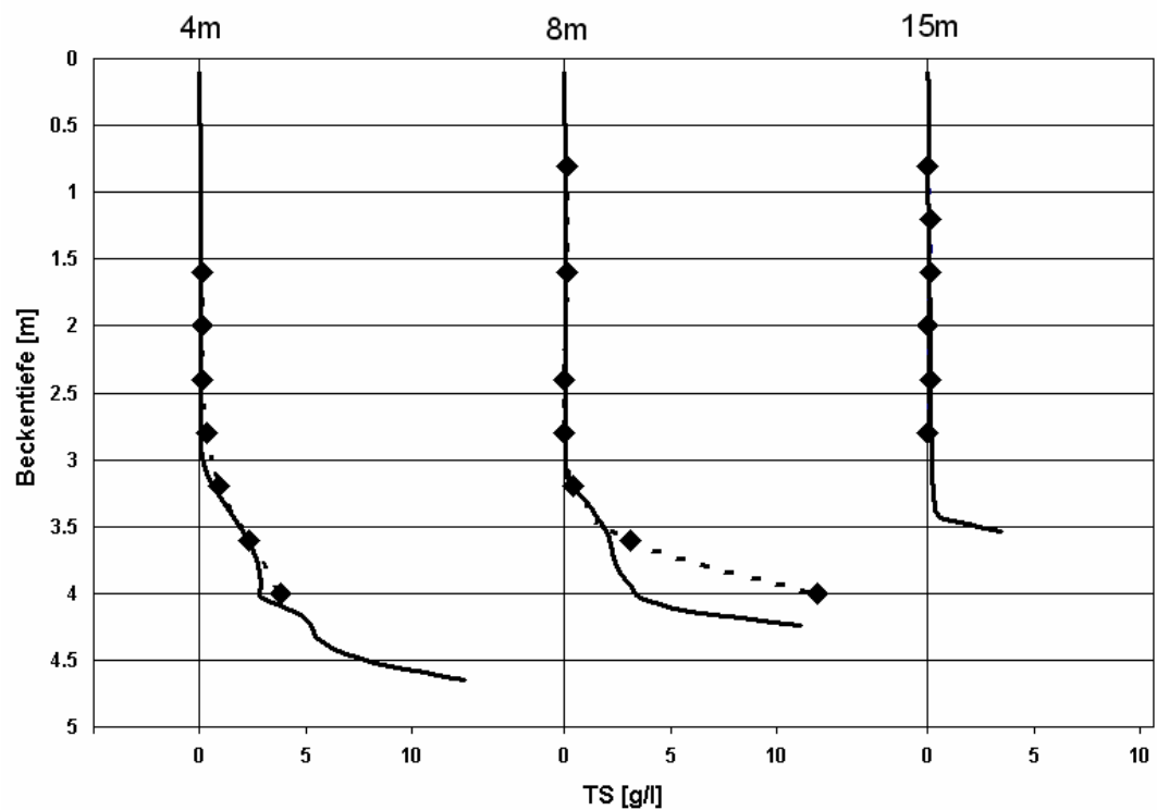
Abbildung 5.44: Vergleich von simulierter und gemessener Schlammverteilung
