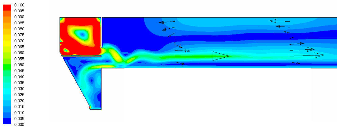
Abbildung 5.32: Geschwindigkeitsverteilung [m/s] – Einlaufbereich – Optimierung
