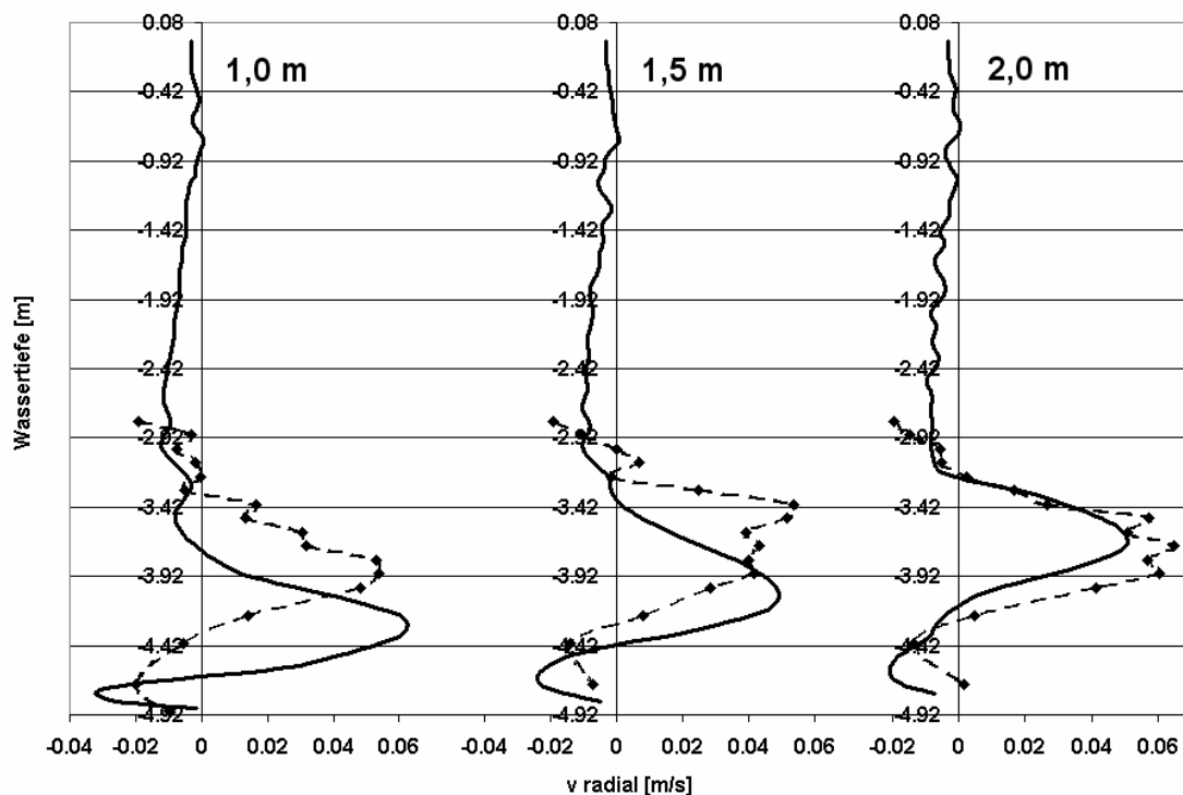
Abbildung 4.9: Vergleich von gemessenen und simulierten Radialgeschwindigkeiten – hoher Einlauf – Lastfall 1
