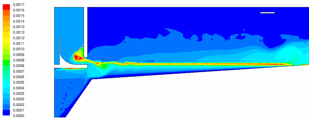
Abbildung 4.18: Verteilung der Sinkgeschwindigkeit [m/s] - tiefer Einlauf
