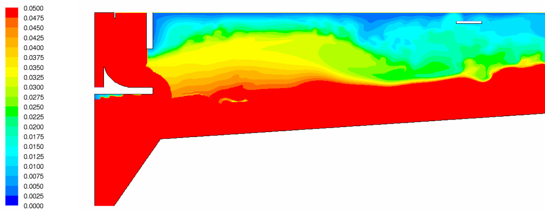
Abbildung 4.5: Schwebstoffverteilung [g/l] - hoher Einlauf
