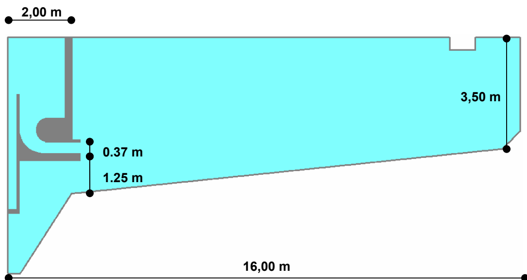
Abbildung 5.46: Querschnitt der Optimierungsvariante 2
