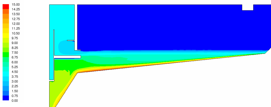
Abbildung 5.49: Schlammverteilung [g/l] – Variante 1
