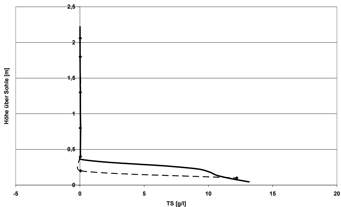
Abbildung 5.13: Vergleich von gemessener und simulierter Feststoffverteilung – 20 m vom Einlauf
