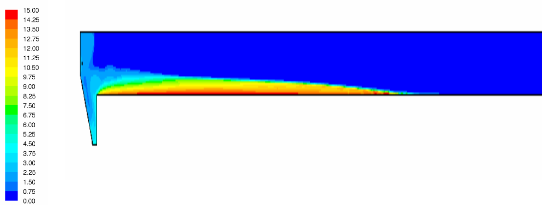
Abbildung 5.24: Schlammverteilung [g/l] – Studie 5
