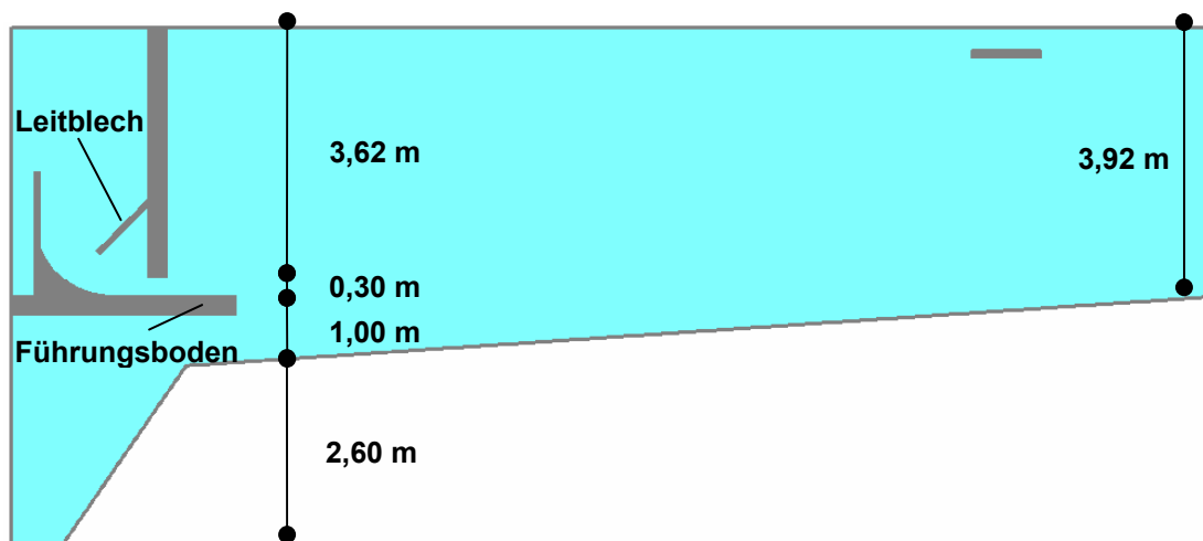
Abbildung 4.26: Querschnitt des Nachklärbeckens Rheda-Wiedenbrück mit optimiertem Einlauf
