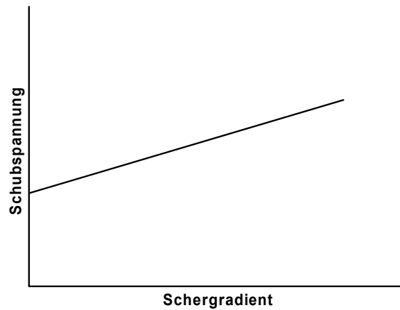
Abbildung 2.5: Scherdiagramm eines idealen Bingham-Mediums
