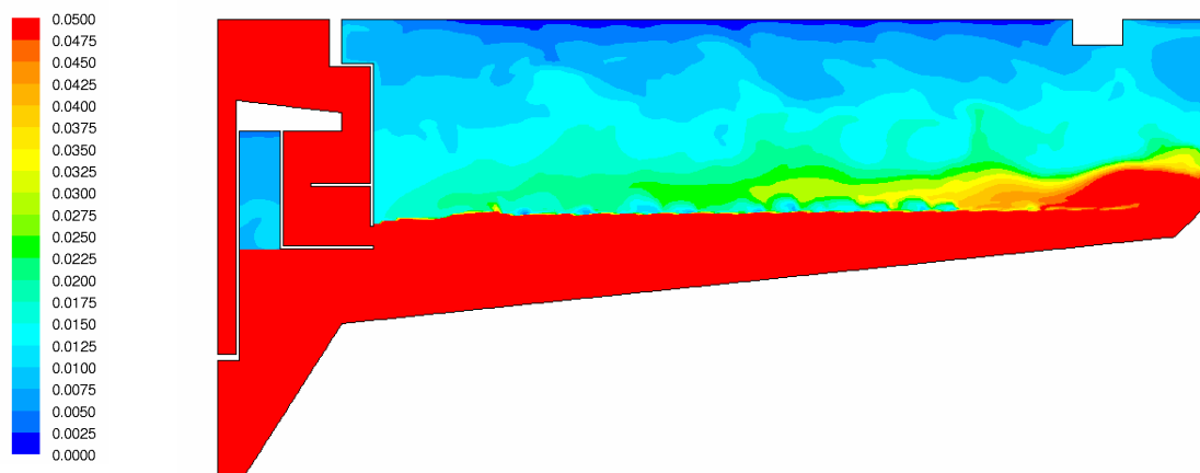
Abbildung 5.56: Schwebstoffverteilung [g/l] – Variante 3
