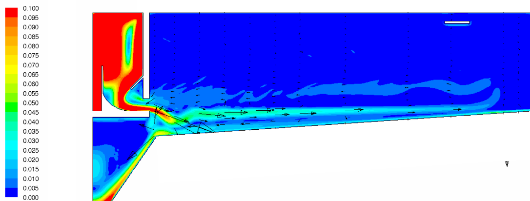
Abbildung 4.15: Geschwindigkeitsverteilung [m/s] - tiefer Einlauf
