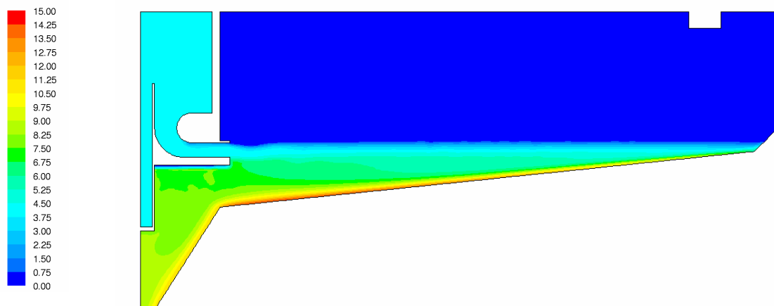
Abbildung 5.52: Schlammverteilung [g/l] – Variante 2
