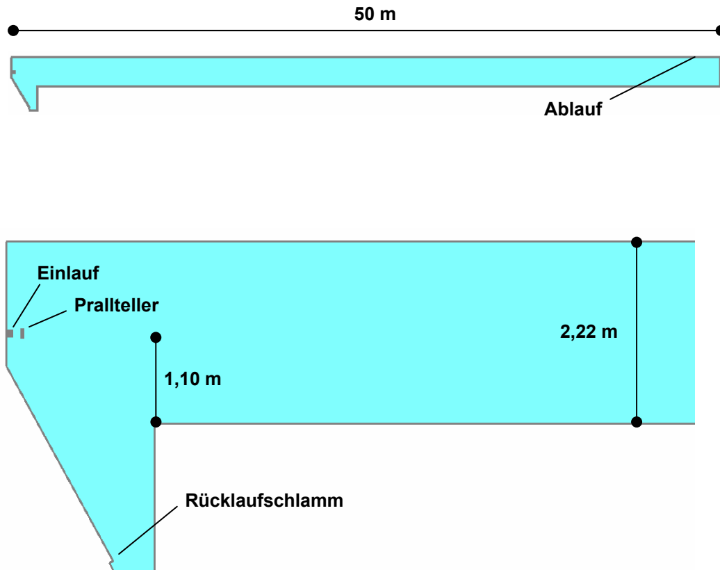
Abbildung 5.1: Schnitt durch das Nachklärbecken der Kläranlage Kierspe
