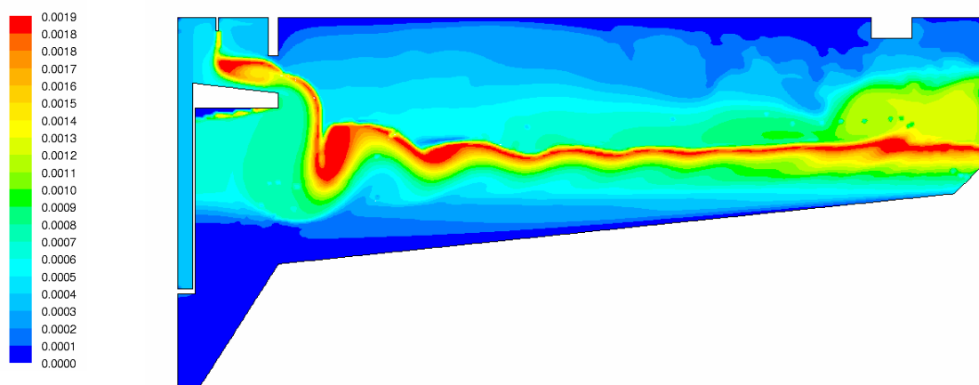
Abbildung 5.41: Verteilung der Sinkgeschwindigkeit [m/s]
