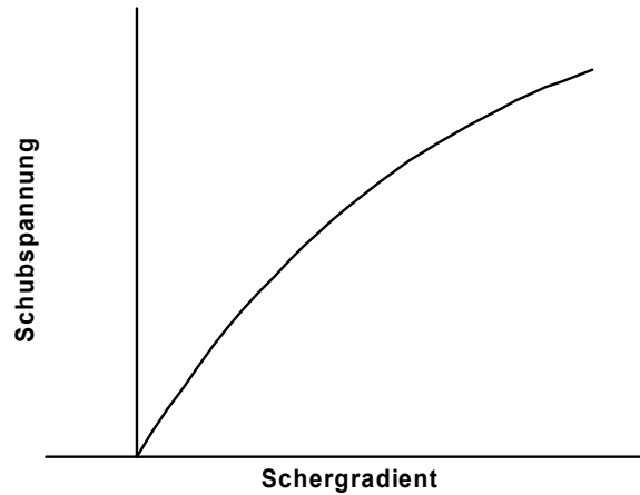
Abbildung 2.4: Fließkurve von strukturviskosen Medien
