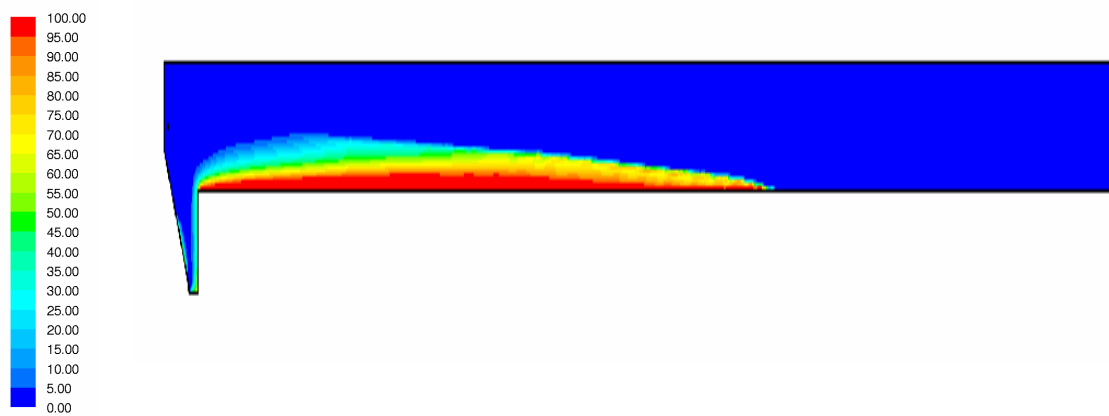
Abbildung 5.23: Verteilung der Viskosität [Ns/m²] – Studie 4
