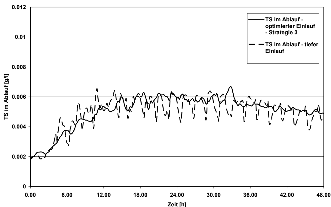
Abbildung 4.37: Simulierte TS-Konzentrationen im Ablauf der Nachklärbecken bei konstanter Beschickung von 140 \text{ m}^3/15\text{min} .
