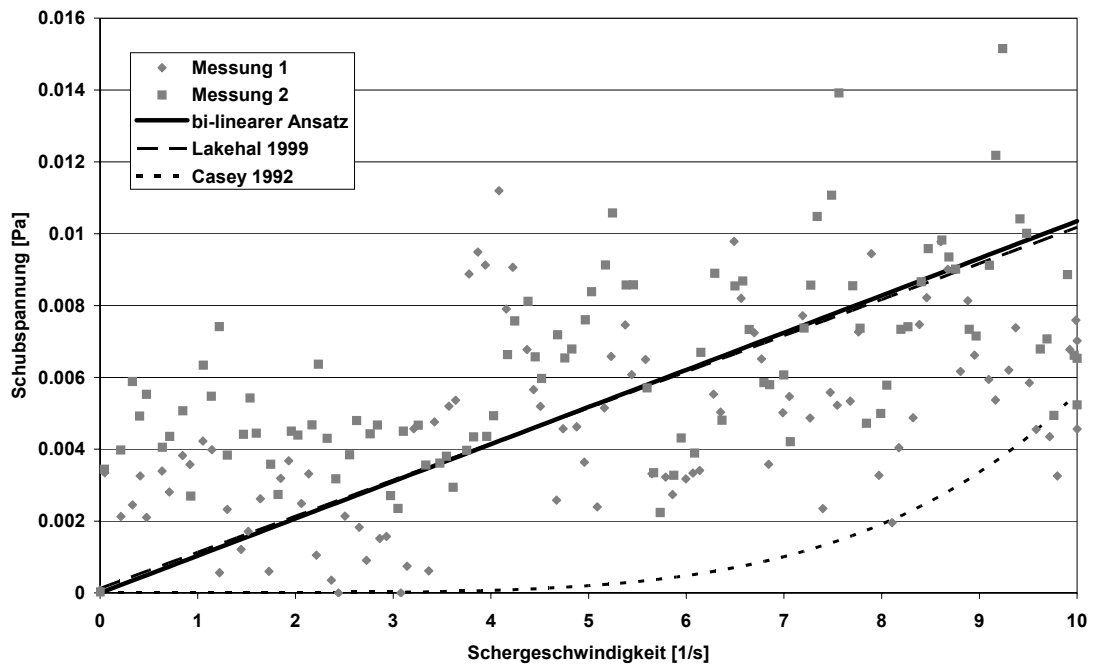
Abbildung 3.7: Schubspannungen bei einer TS-Konzentration von 0,1 g/l
