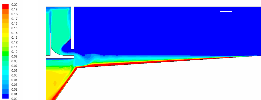
Abbildung 4.19: Verteilung der Viskosität [Ns/m²] - tiefer Einlauf
