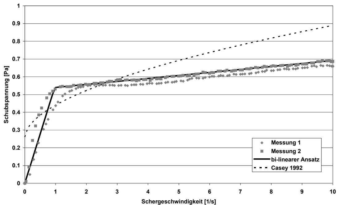
Abbildung 3.13: Schubspannungen bei einer TS-Konzentration von 12,6 g/l
