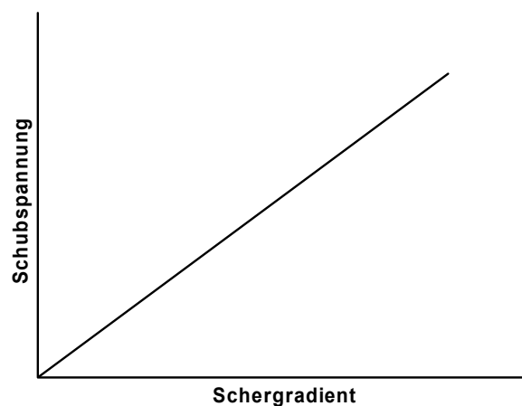
Abbildung 2.3: Scherdiagramm eines newtonschen Fluides
