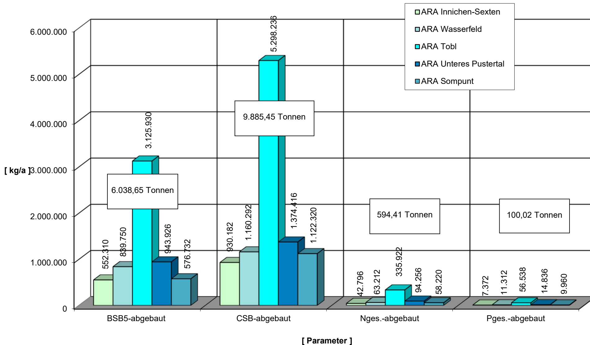
Vergleich der abgebauten Schmutzfrachten in kg pro Jahr; Jahr 2025
