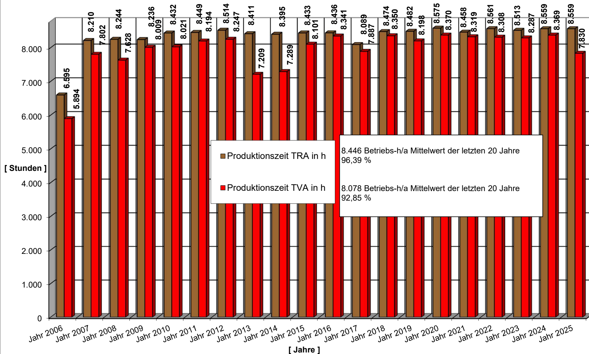
Produktionszeit der thermischen Trocknungs- und -Verwertungsanlage in h; Jahre 2006-2025
